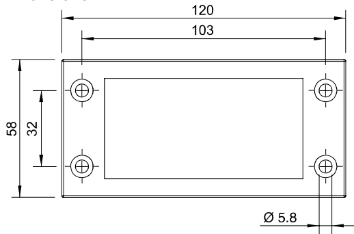
外形尺寸 Dimensions
