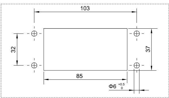
开孔尺寸 Cut-out
