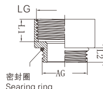
圆形金属扩径环 Round metal enlargement
