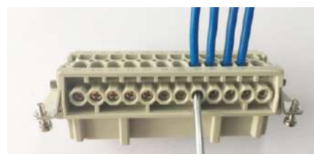
Step 4:连接完成，请拉动线缆以确认线缆确实被弹片夹紧。
