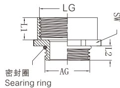
六角金属扩径环 Hexagonal metal enlargement
