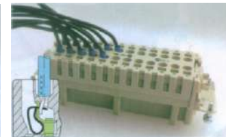
Step 4:连接完成，请拉动线缆以确认线缆确实被弹片夹紧。
