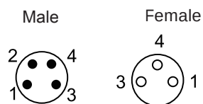
M8Male
