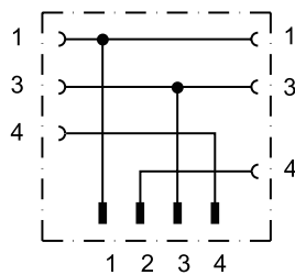
M8Male
