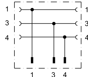
M8Male
