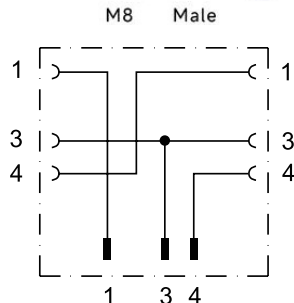
M8Male
