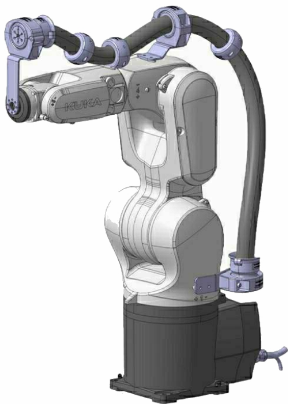
FA-KUKA-KR6-R700-ARC-1-6A
