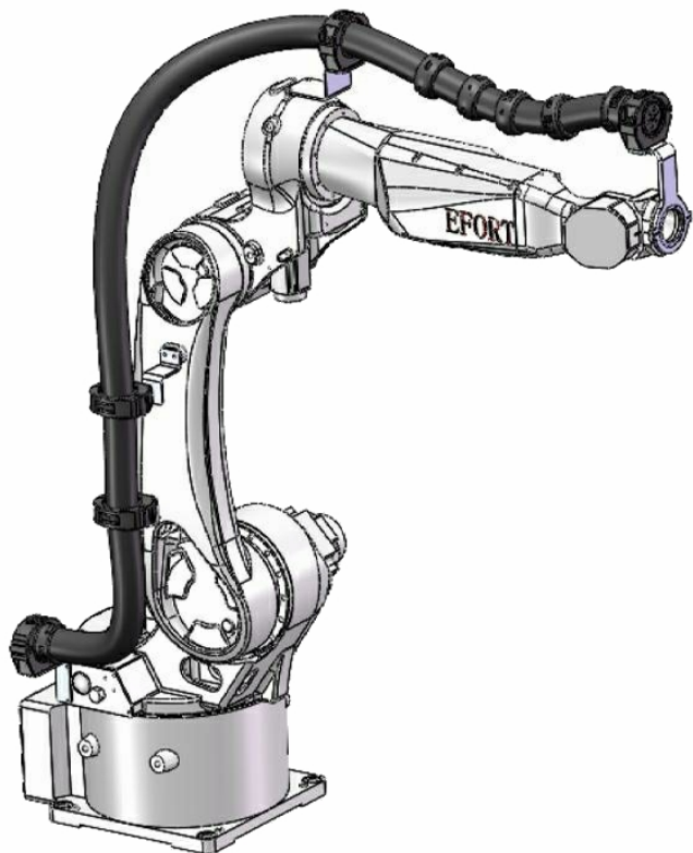
FA-EFORT-ARCQO-1600-ARC-1-6A
