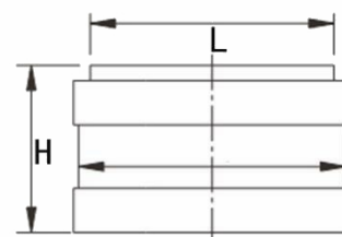
DL-RGFX-56/70A
