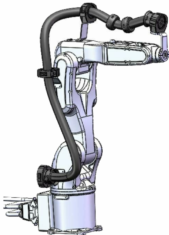
FA-EFORT-ER7-900-ARC-1-6A
