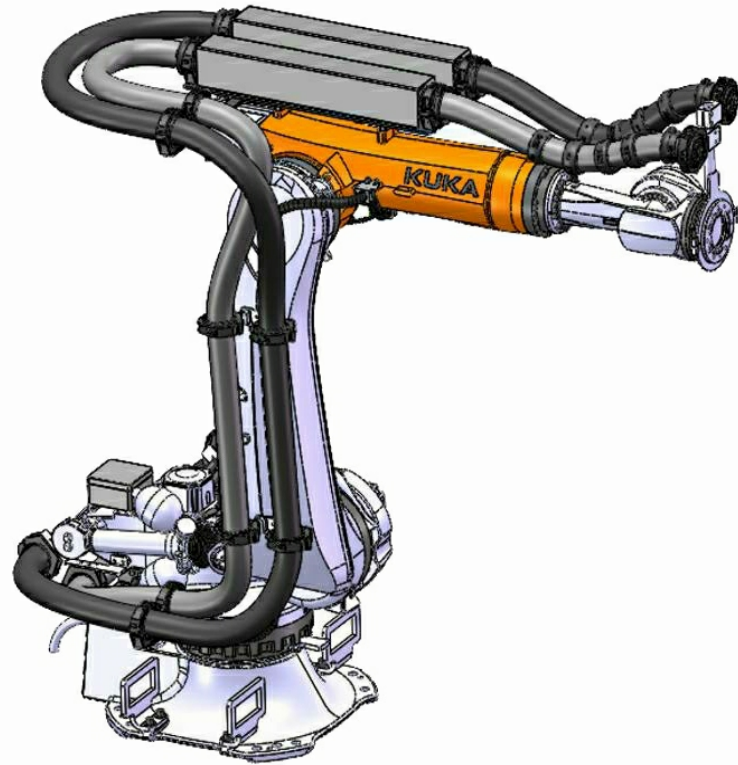
FA-KUKA-KR300-R2700-MH-1-6A
